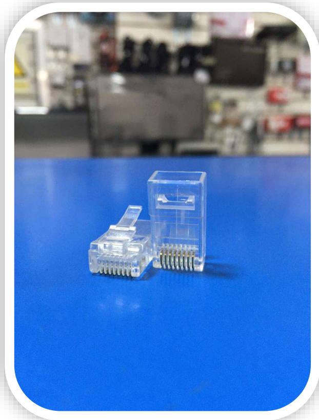
RR-TMP8. Conector RJ45 Nexxt, Categoría 5e
